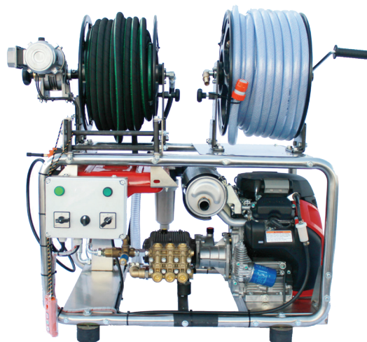
ביובית 24 כ"ס 50 ל/ד 150 באר
